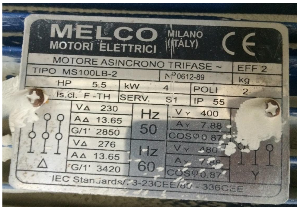
Slika 3.21. Natpisna pločica motora otprašivača
