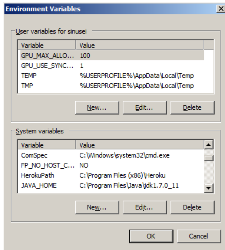
Slika 3.3: „Varijable okruženja“
