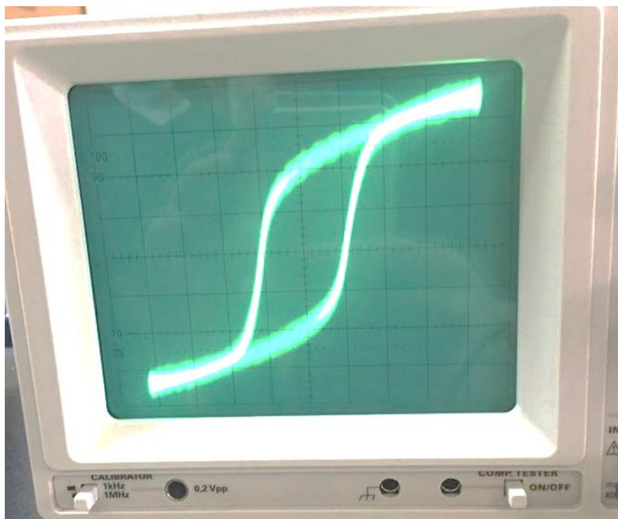
Sl. 4.2. Petlja histereze ponovno namotanog transformatorja
