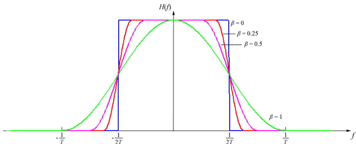
Sl.2.5. Prijenosna karakteristika filtra sa kosinusnim zaobljenjem [7]
