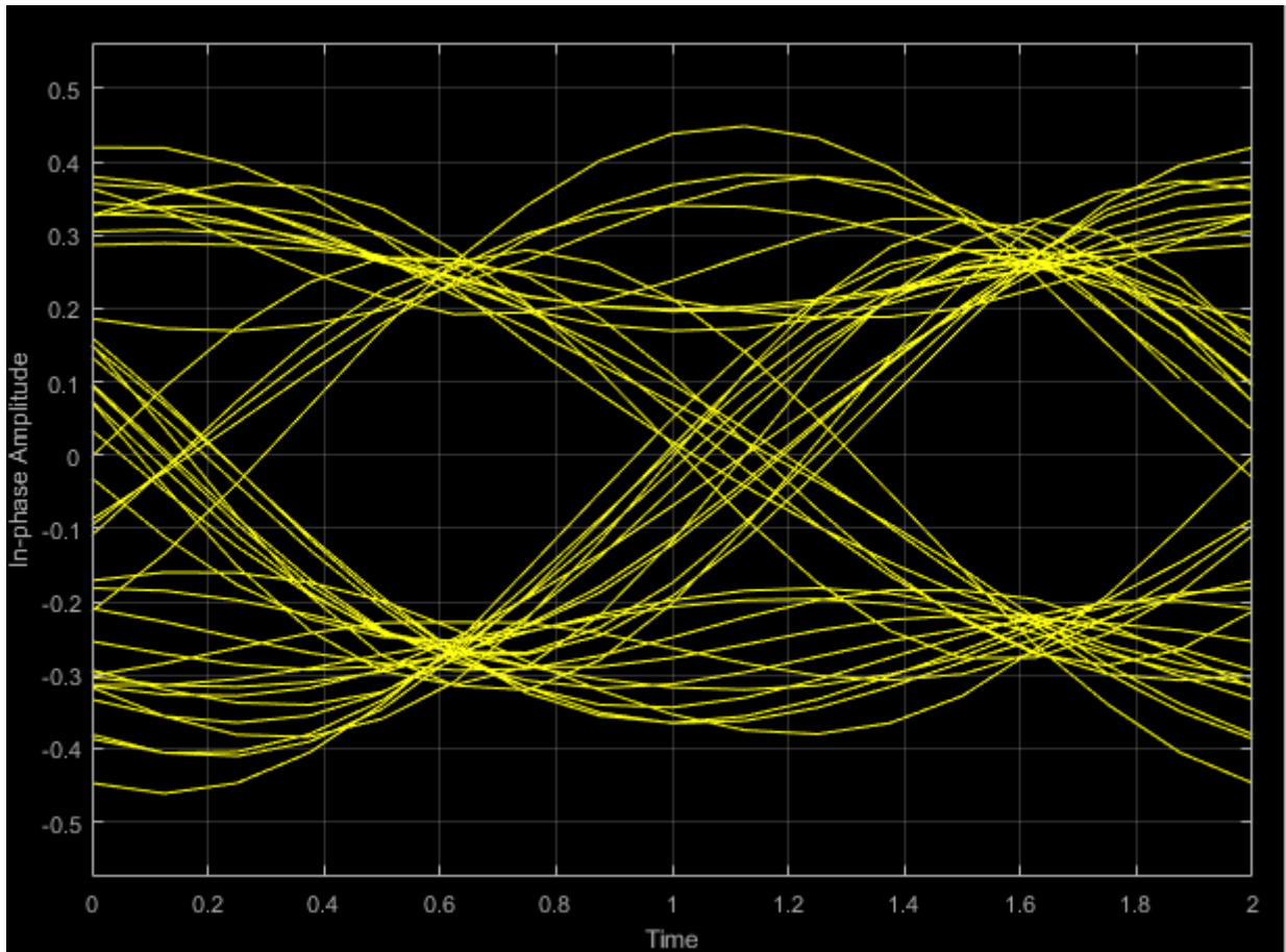
Sl.3.8. Dijagram oka nakon QPSK
