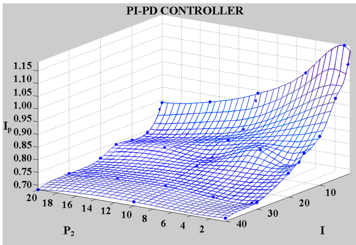
Sl. 5.11. Indeks performansi za PI-PD regulator. [8]
