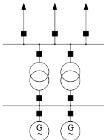
Slika 2.18. Shema spoja generatora na mrežu višeg napon
