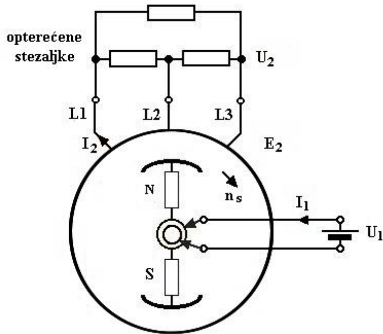
Slika 3.7. Opterećeni generator [14]
