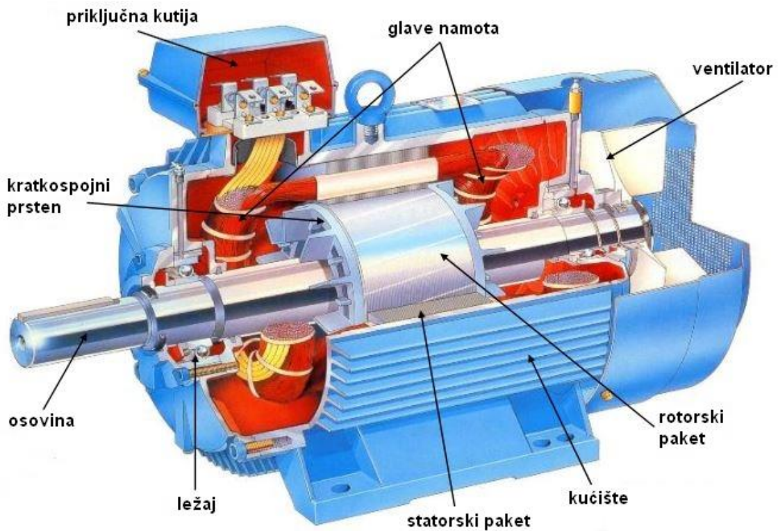
Slika 2.17. Asinkroni stroj [11]
