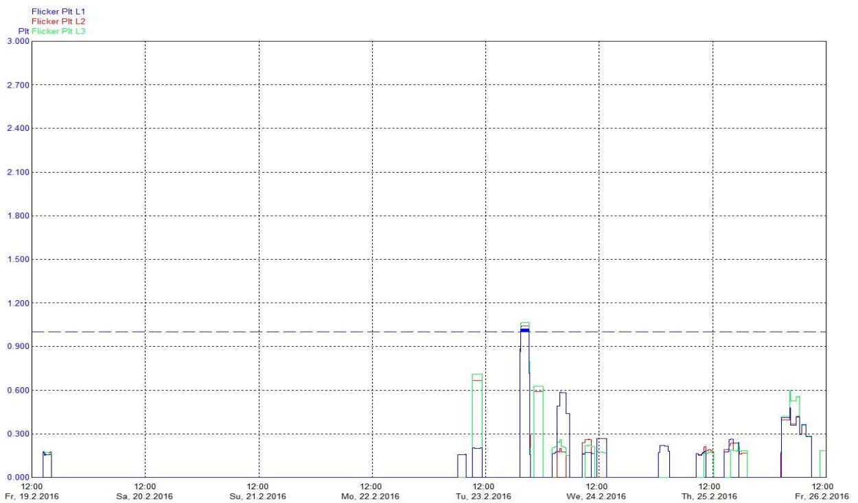
Slika 8.5. Dugotrajno naponsko treperenje (flikeri), prije priključenja BPP.
