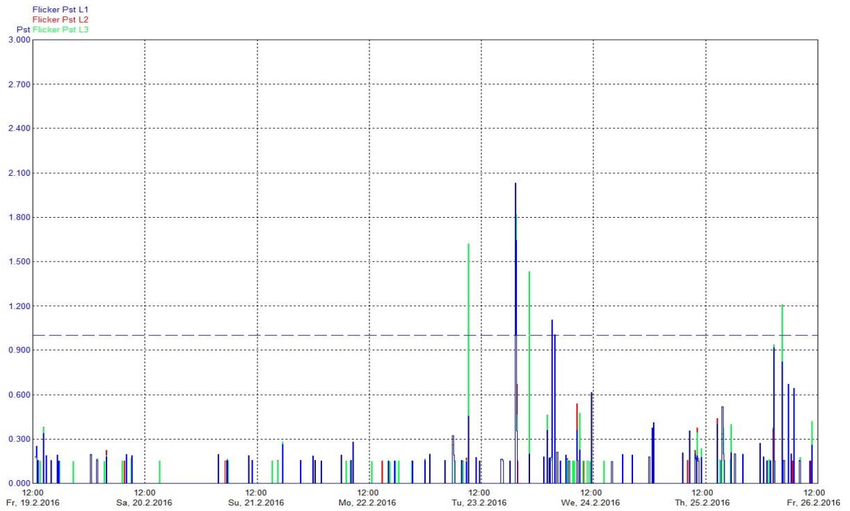
Slika 8.4. Kratkotrajno naponsko treperenje (flikeri) prije priključenja BPP.
