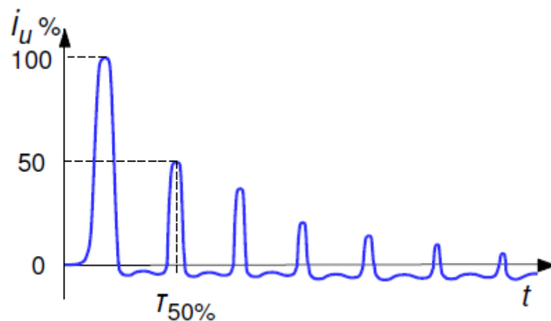
Slika 2.1. Struja uklapanja [2]
