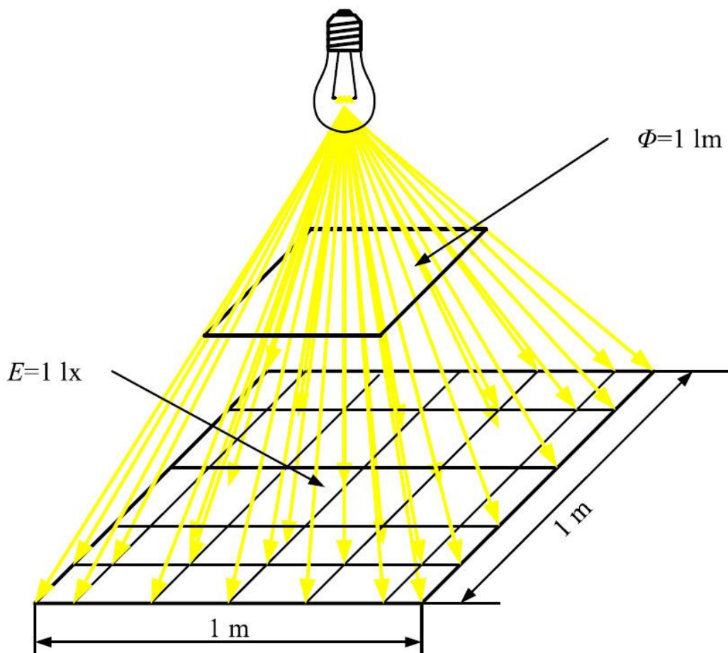
Slika 3.3. Definicija jedinice za rasvjetljenost
