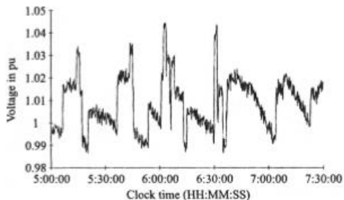
Slika 3.10. Kratkotrajni previsoki napon[9]
