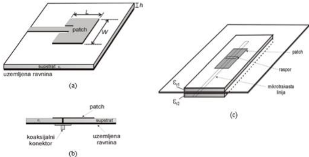
Slika 3.2. Pobude mikrotrakaste antene na uzemljenoj podlozi a) pobuda pomoću mikrotrakaste linije ; b) pobuda pomoću koaksijalne linije ; c) pobuda pomoću raspore
