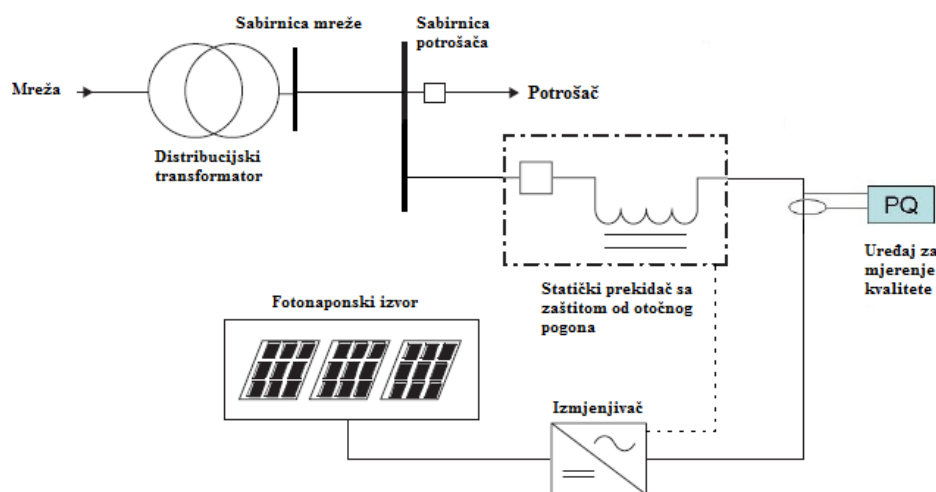
Sl. 5.1. Principijelna shema fotonaponske elektrane.
