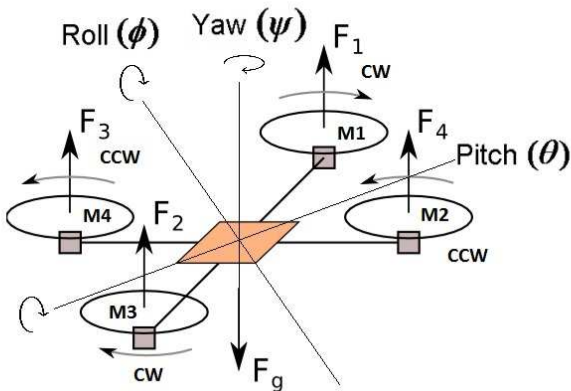
Slika 2.2.2 Osi rotacije i sile na letjelici[7]
