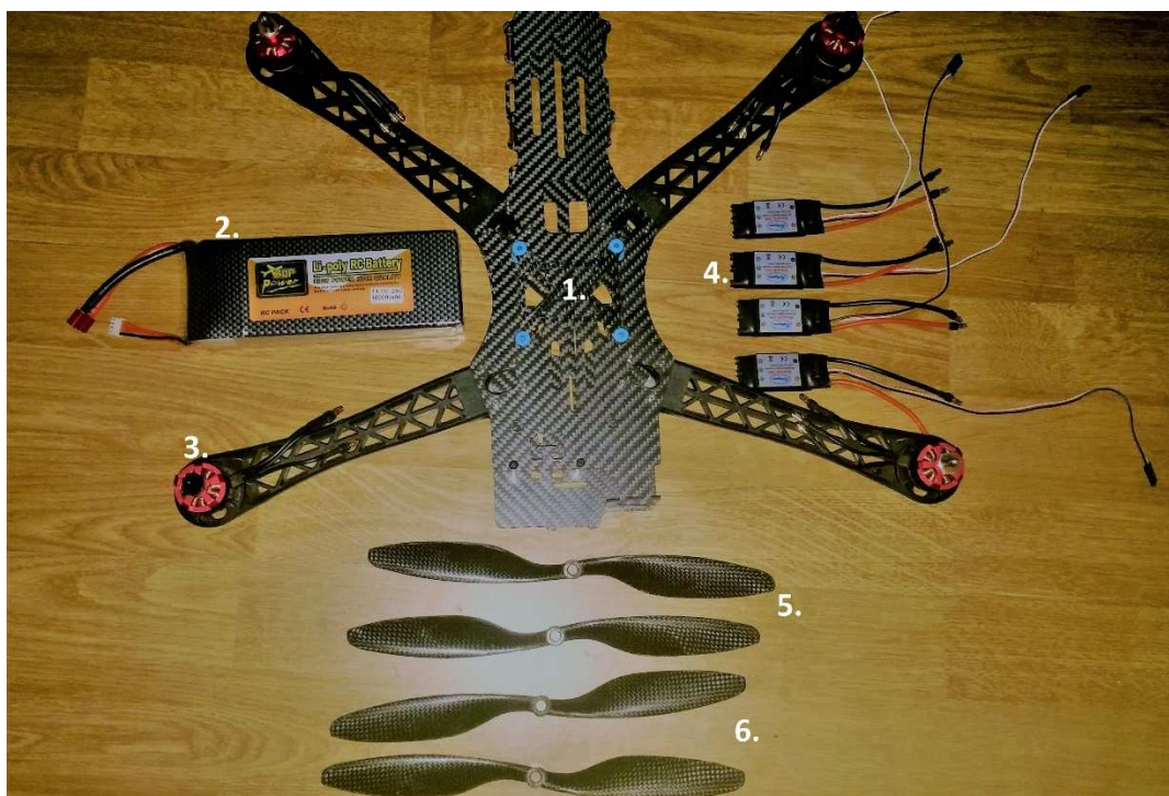
Slika 3.2.1.11. Dijelovi letjelice
