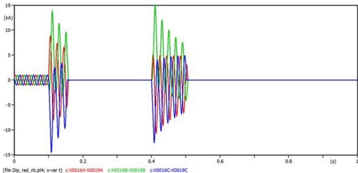
Sl. 5.13. Valni oblici struja pojedinih faza generatora pri trofaznom kratkom spoju
