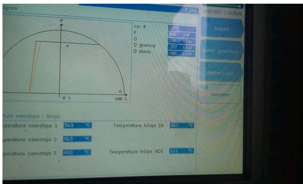
Slika 5.21. P/Q dijagram generatora
