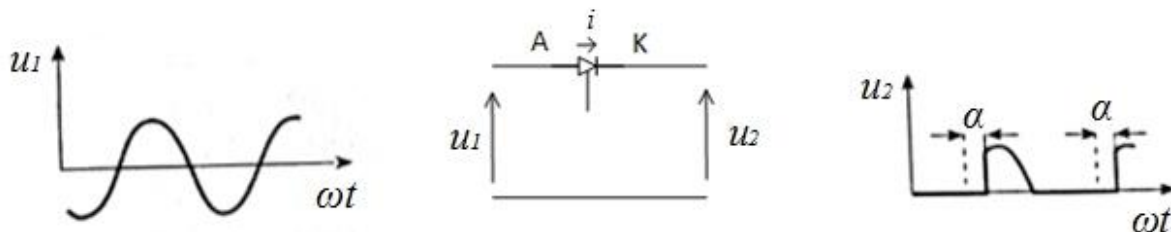
Slika 2.9. Tiristor [1]
