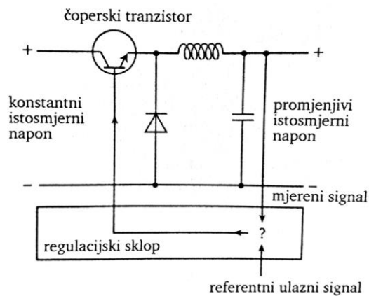
Slika 2.22. Regulacija napona napajanja u istosmjernom međukrugu [1]
