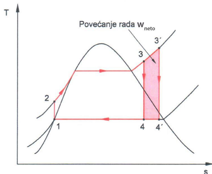
Slika 2.13. Povišenje temperature pregrijane pare (T-s dijagram) [10]
