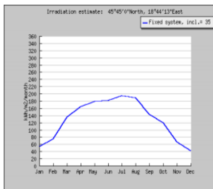
Mjesečno Sunčevo zračenje pod fiksnim kutem dobiveno FN sustavom
