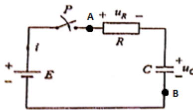
Slika 4 Shema spoja
