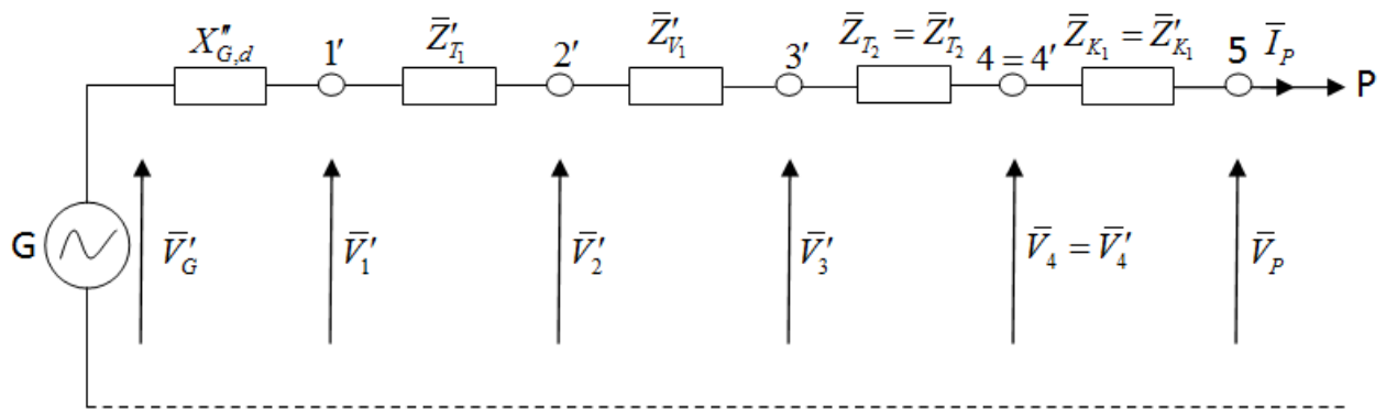
Sl. 5.3. Nadomjesna reducirana shema sustava
