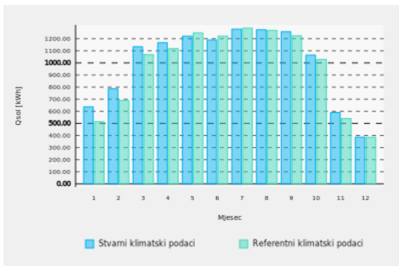
Slika 4.16. Toplinski dobitci od Sunčeva zračenja ( Q_{sol} )
