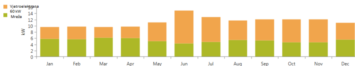
Slika 4.17. Mjesečna prosječna proizvodnja snage od strane vjetroelektrane Bergey Excel 6 kW i distribucijske mreže [24]
