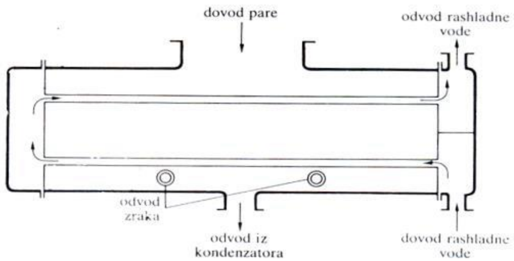
Slika 4.6. Skica kondenzatora [12]
