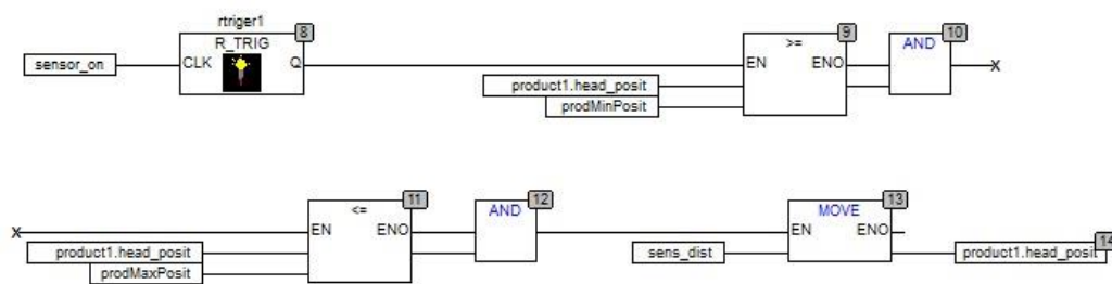
Slika 2.31. Korekcija pozicije.
