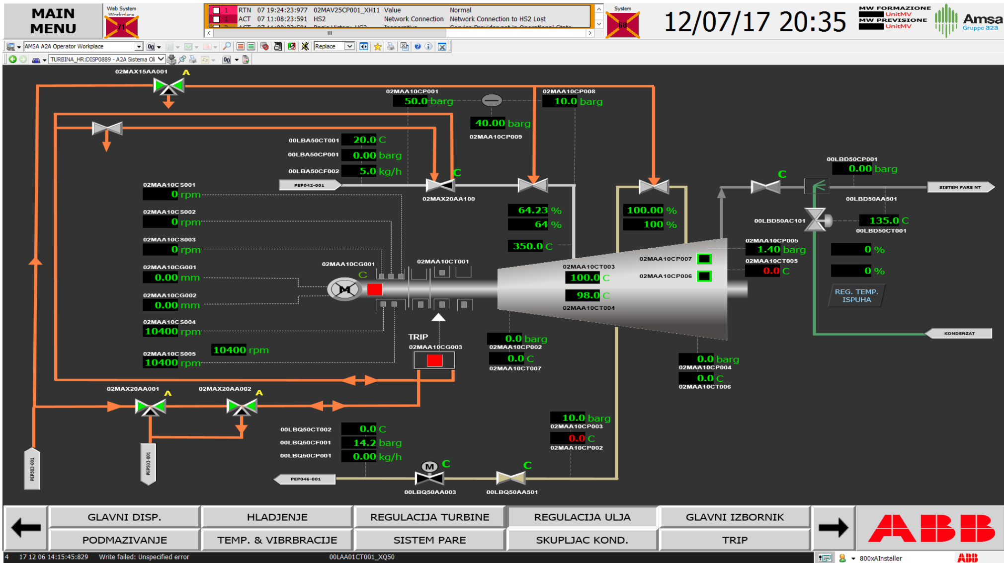
Slika 7.7 Regulacije ulja
