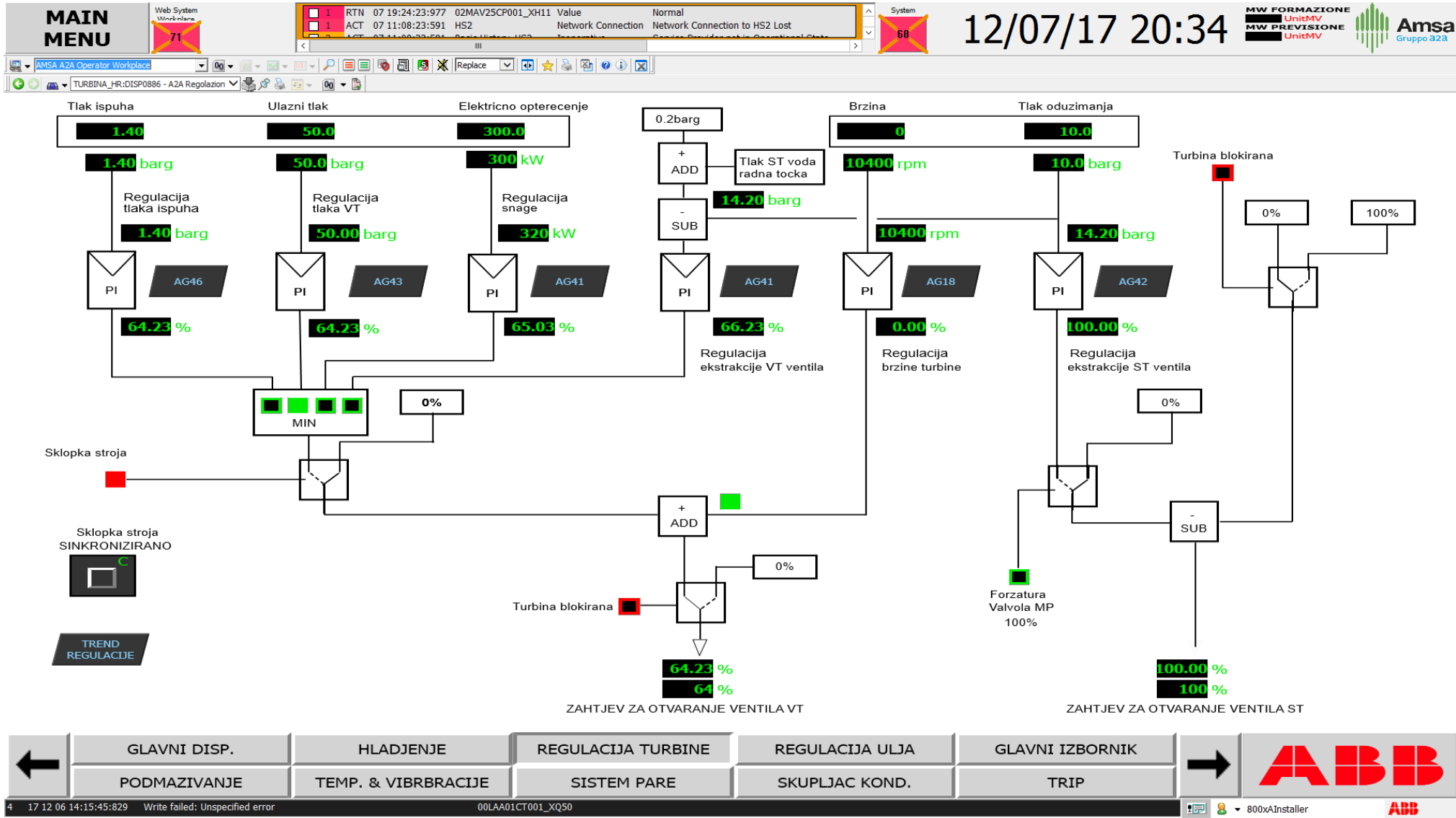
Slika 7.5 Regulacija HMI
