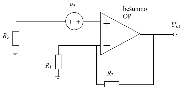
Slika 3.13. Utjecaj šuma napona u_{\delta} na izlazni napon U_{izl}
