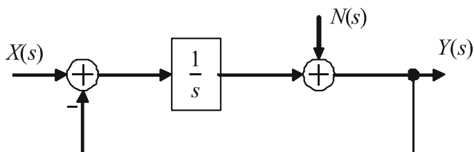
Slika 2.3. Sigma-delta modulator prvog reda u frekvencijskoj domeni
