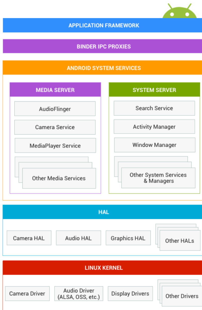
Slika 5. Android arhitektura [15]
