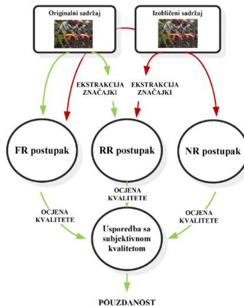
SI.2.12: Metode objektivnih mjerenja kvalitete vizualnog sadržaja, preuzeto iz [26].
