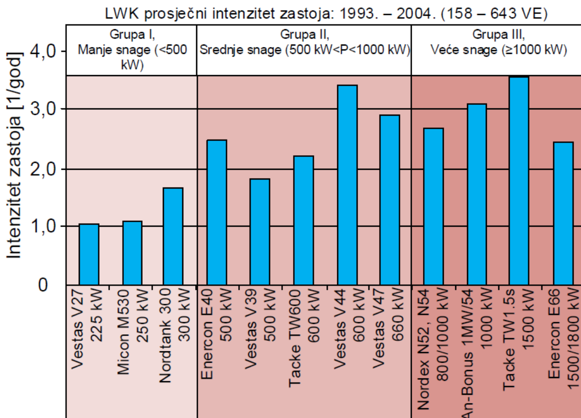
Slika 4.19: Intenzitet zastoja različitih modela, različitih veličina vjetroagregata. Preuzeto iz (Topić, 2014).
