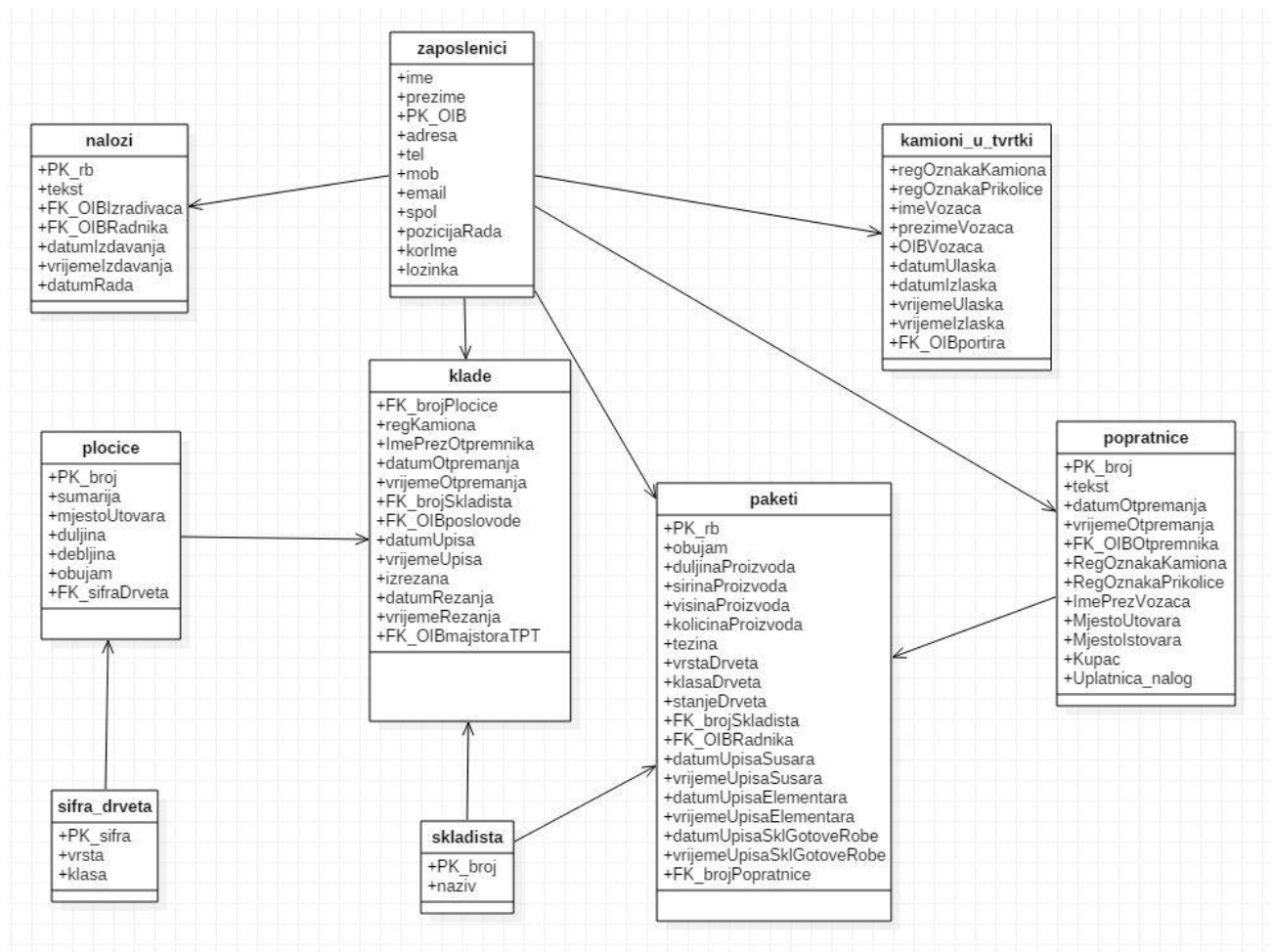
SI. 5.1. UML dijagram baze podataka BazaPodatakaZavrnsniRad
