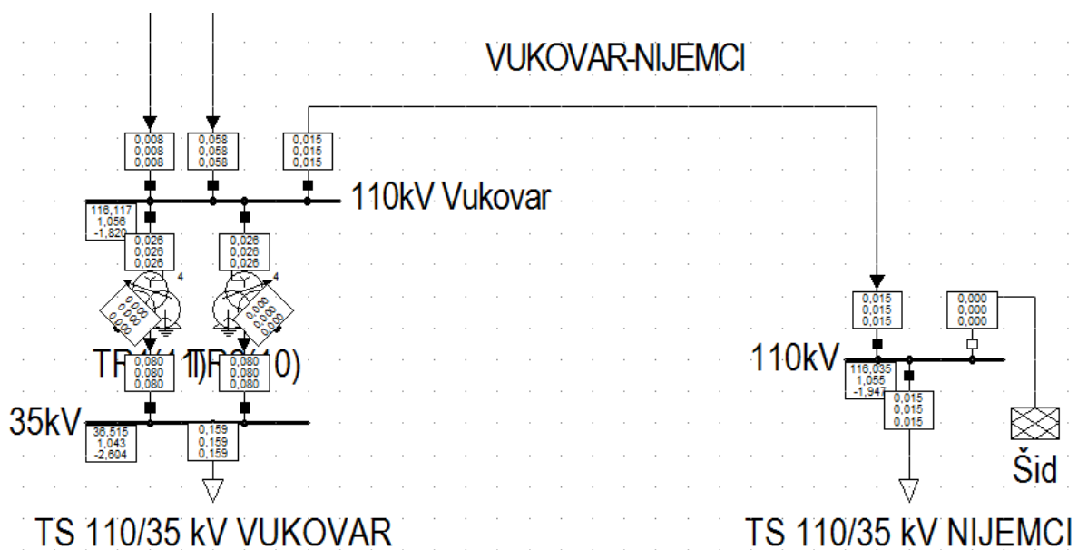
Slika 5.7. Struje u normalnom pogonu pri otpjenoj nadomjesnoj mreži "Šid"
