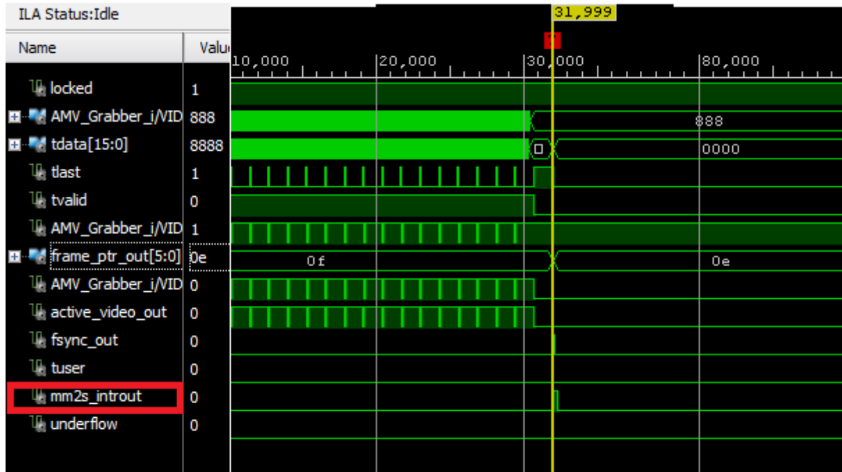
Sl. 5.3 ILA podaci uhvaćeni pod uvjetom da se signal mm2s_introut dogodio.
