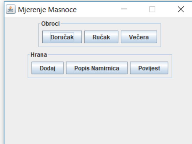
Slika 3.1. Glavni prozor.
