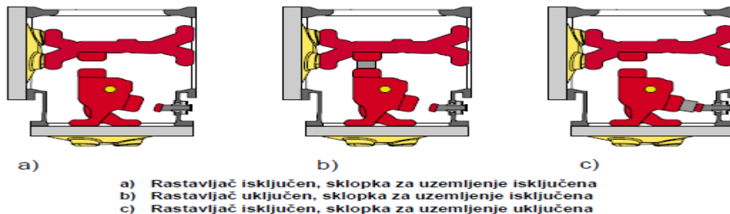
Sl.3.4. Uklopni položaji rastavljača i sklopke za uzemljenje [2]
