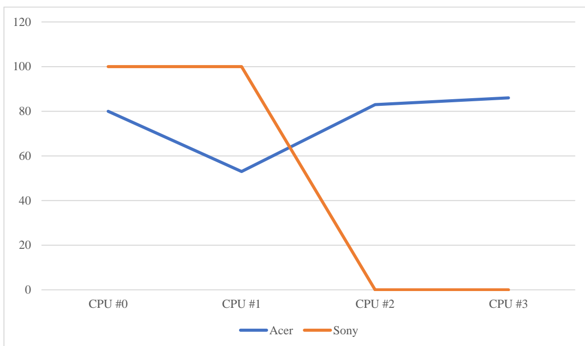
Grafikon 5.4. HeavyLoad CPU iskorisštenost (dvije jezgre)
