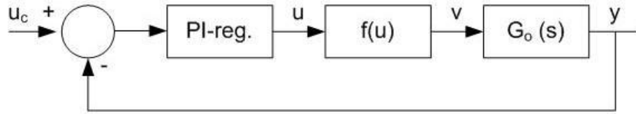
Sl. 3.4. Blok prikaz promatranog regulacijskog kruga s izraženim nelinearnim regulatorom
