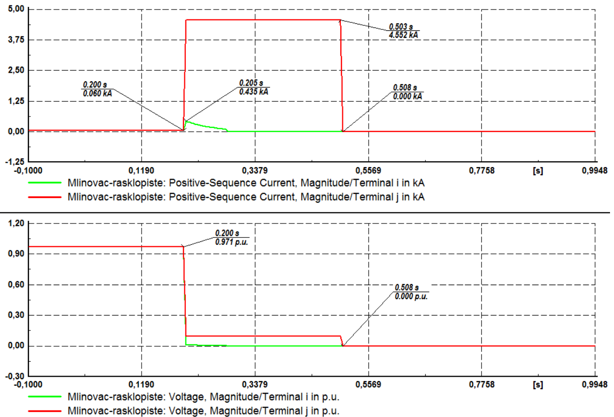
Slika 4.19. Strujno naponske prilike na vodu Mlinovac-Rasklopište
