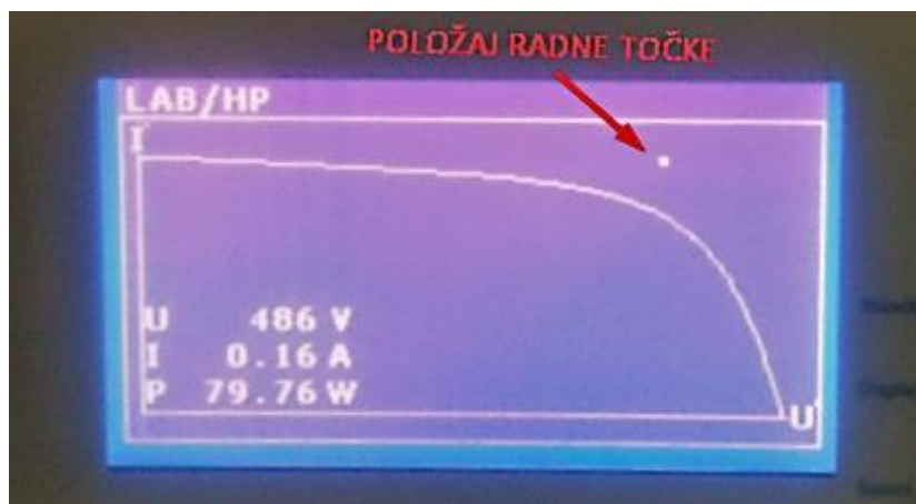
Slika 3.7. Položaj radne točke izvan karakteristike[3]
