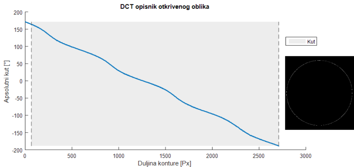
Slika 3.15. DCT opisnik okruglog poklopca
