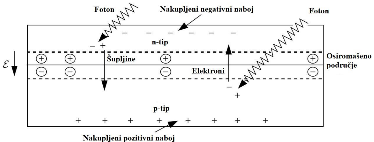
Slika 3.3 Fotonaponska ćelija [9]
