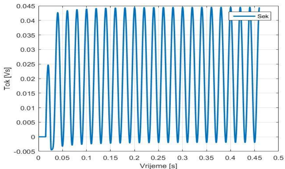
Sl. 3.15. Magnetski tok pri U_m = -36 V i \alpha = 90^\circ .
