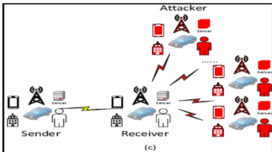
Slika 4.1.3. DDoS napad [11]
