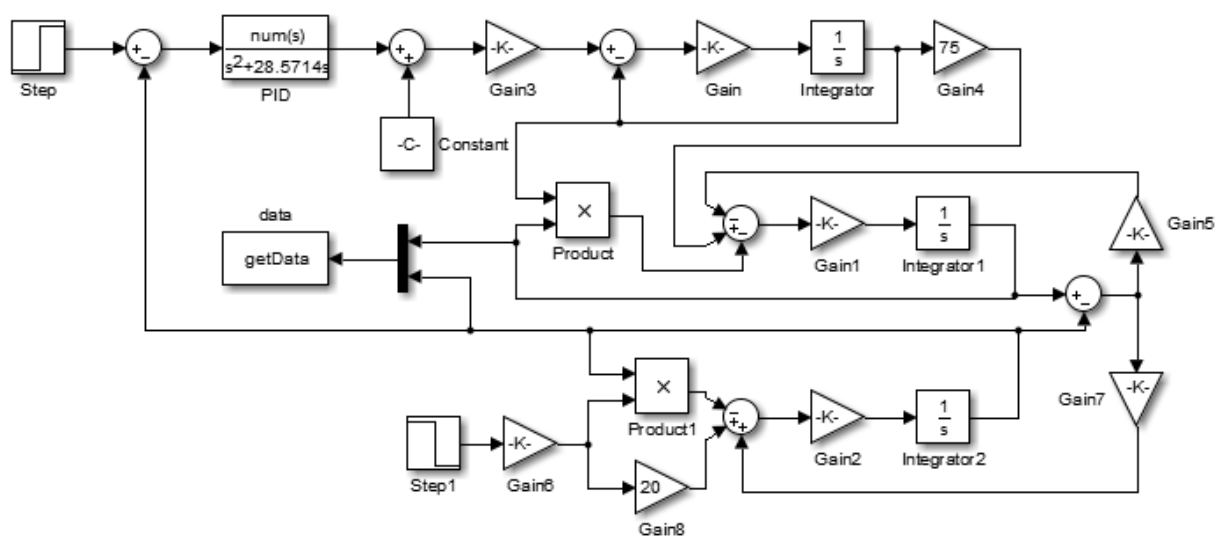
Sl. 3.1. Shema nelinearnog modela sustava upravljanja toplinskim izmjenjivačem
