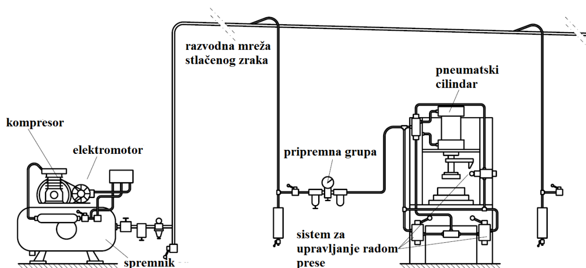
Slika 5.5 – Pneumatski sistem
