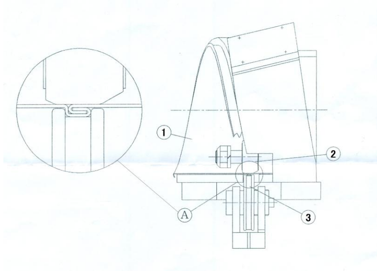
Slika 3.6 - Spojni šav
