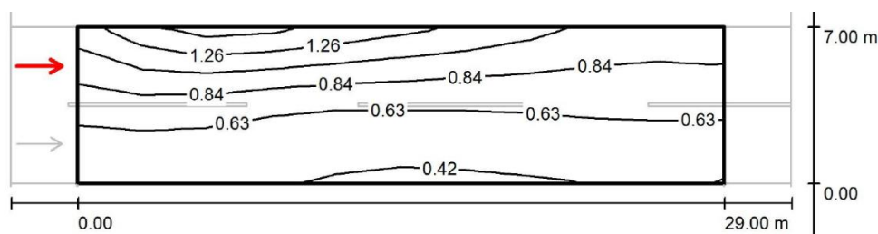
Slika 42. Proračun luminacije za promatrača na lijevoj strani kolnika (bliža rasvjeti)[72]
