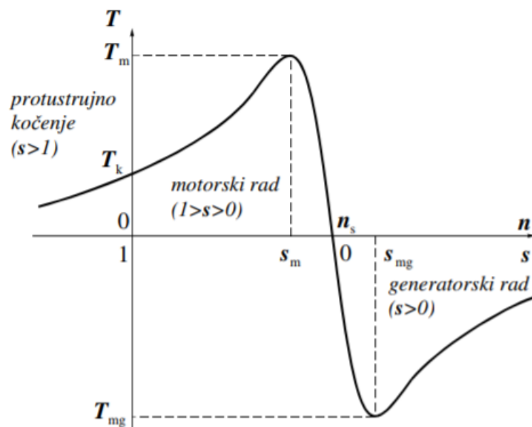
Sl. 2.4: Momentna karakteristika [1]
