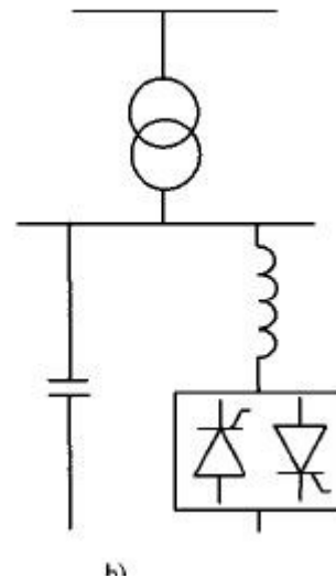
Slika 3.2. Tiristorski kontrolirana zavojnica sa filtrom;[6]
