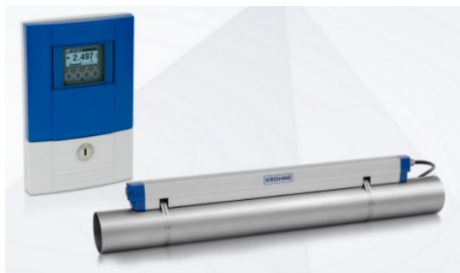
Sl. 4.30. Optisonic 6300 [34]
