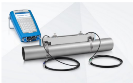
Sl. 4.29. Optisonic 6300 P [33]
