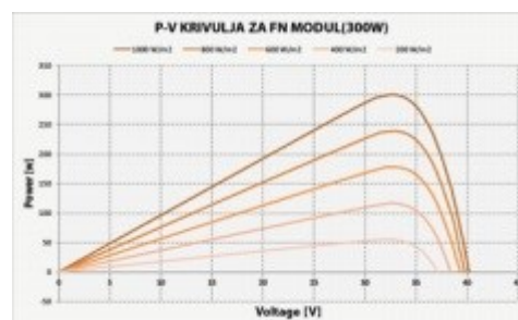
Slika 3.4. P-V krivulja
