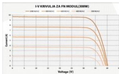
Slika 3.3. I-V krivulja
